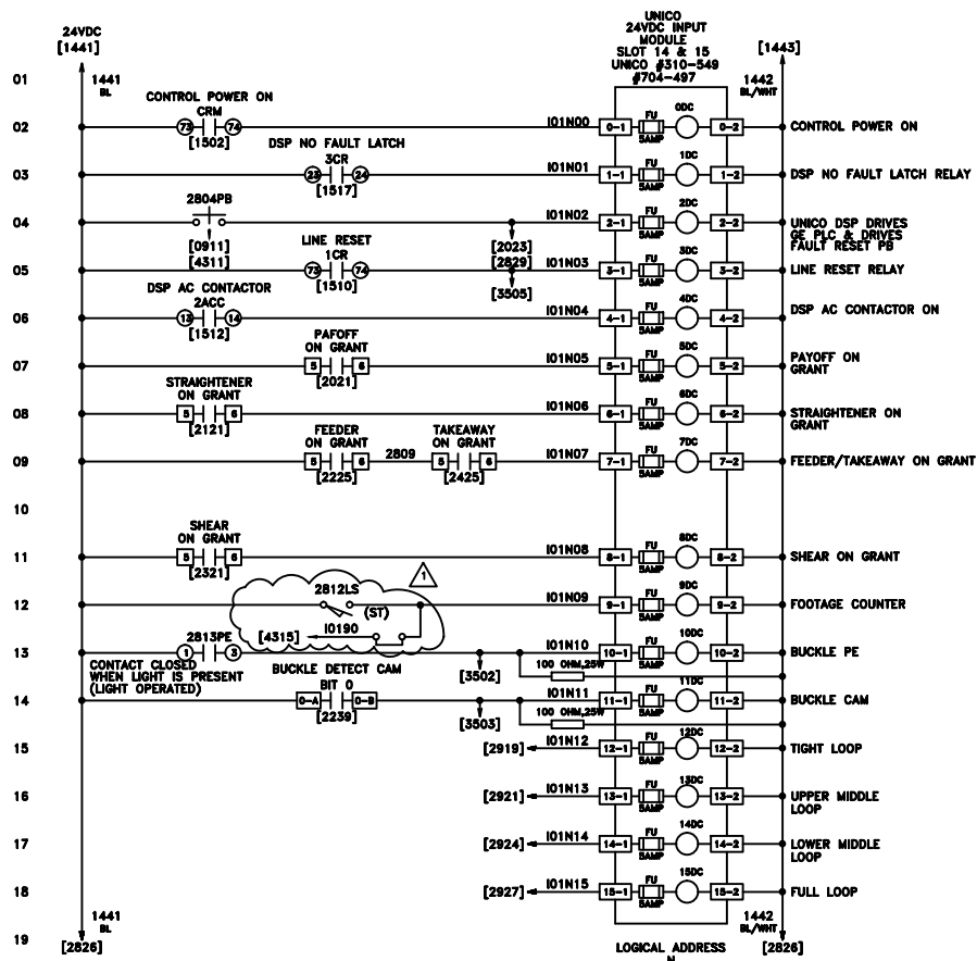
UNICO I/O RACK SLOT N-0
