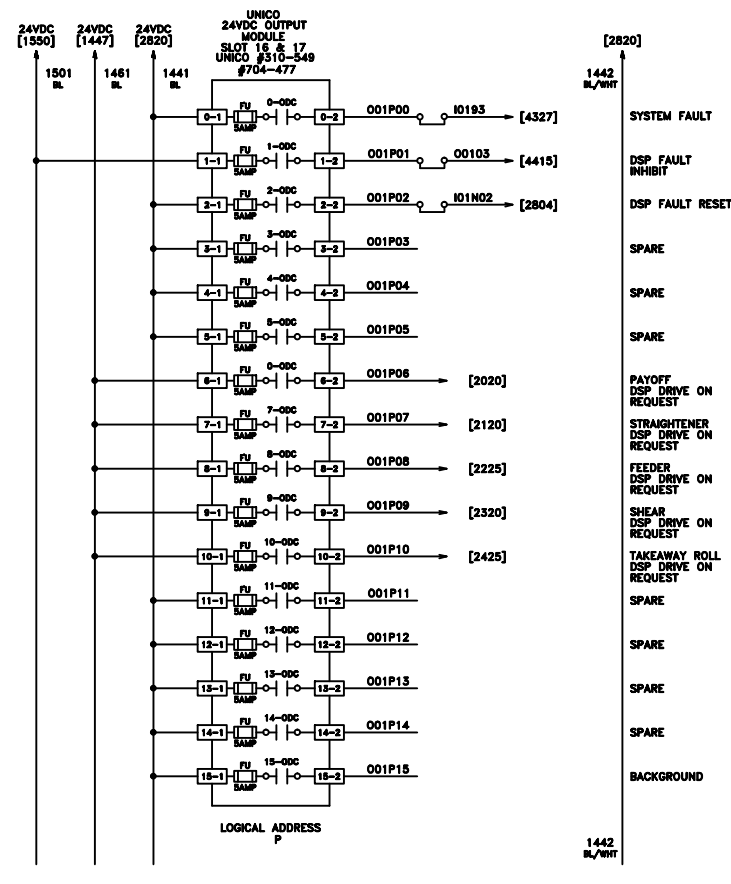
UNICO I/O RACK SLOT P & Q
